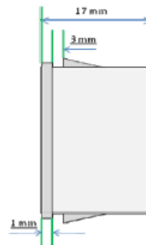
Planta Lateral
