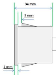
Planta Frontal
